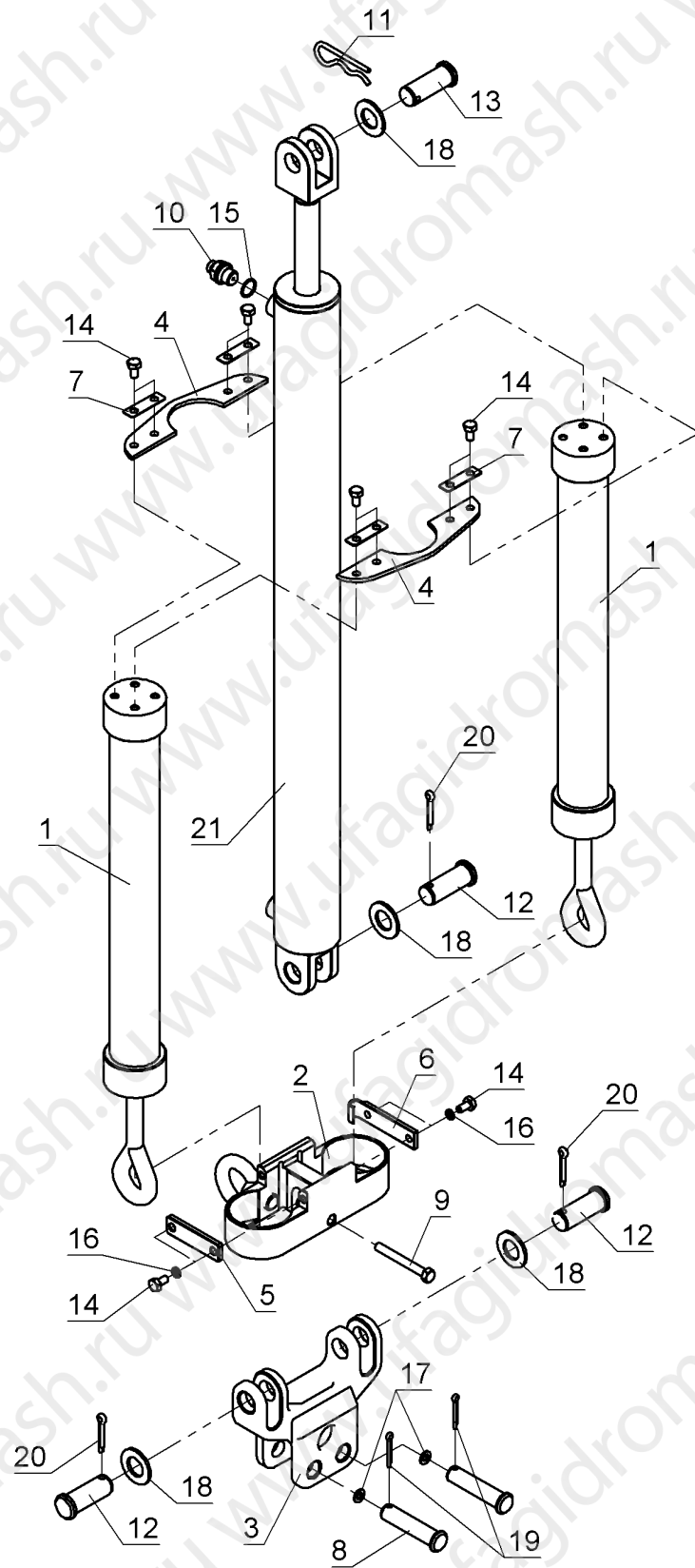
Цилиндр подвески в сборе
