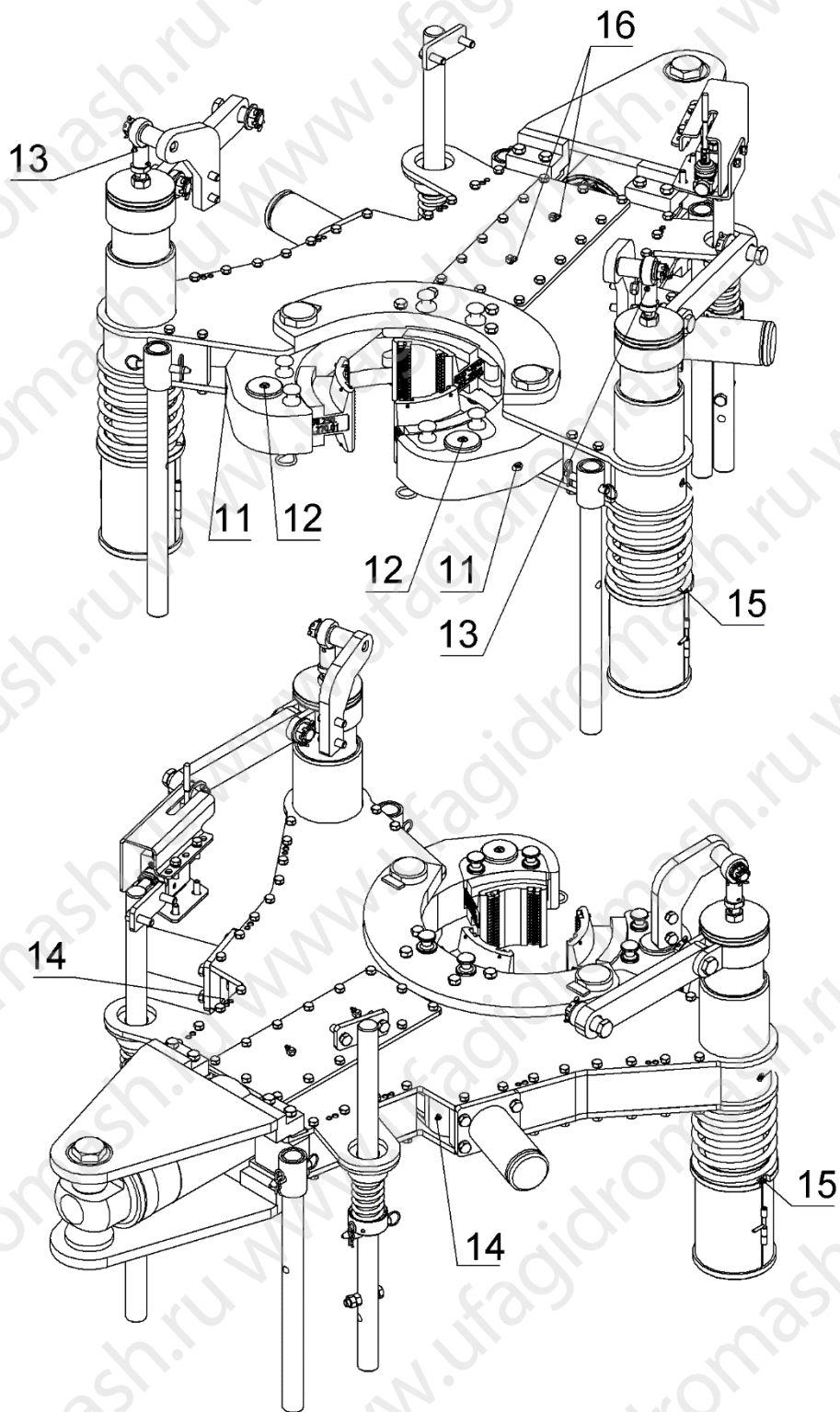
Схема смазки устройства гидравлического стопорного
