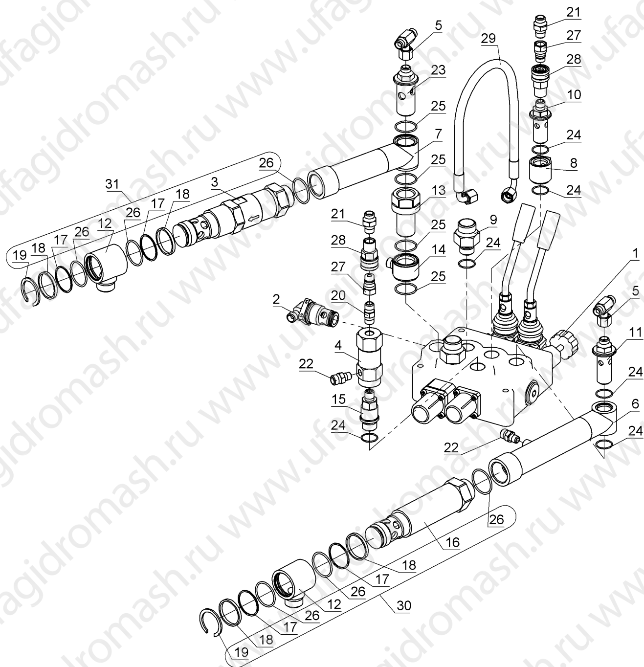
Рисунок 24 Гидро модуль
