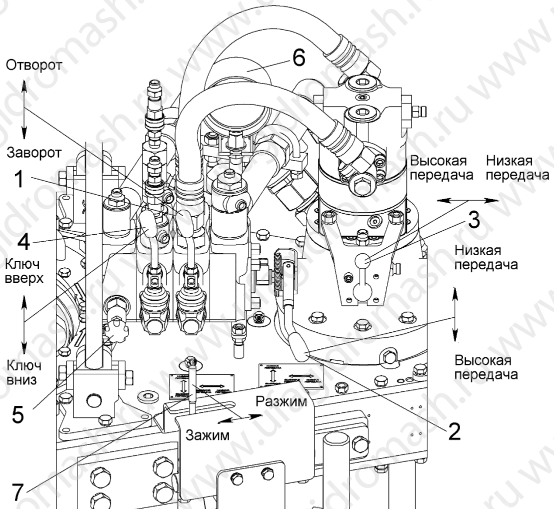
Рисунок 2 Рычаги управления гидроклапа
