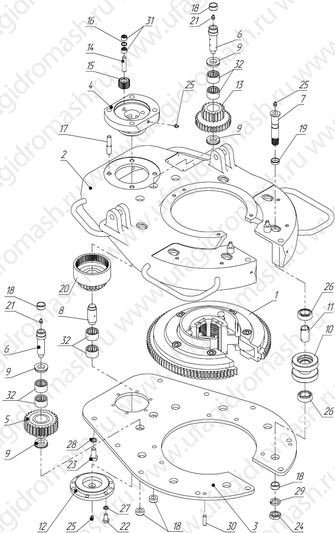
Рисунок 13 Редуктор зубчатый
